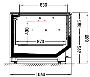
WNEV/WDEV-06-1605G XXX
